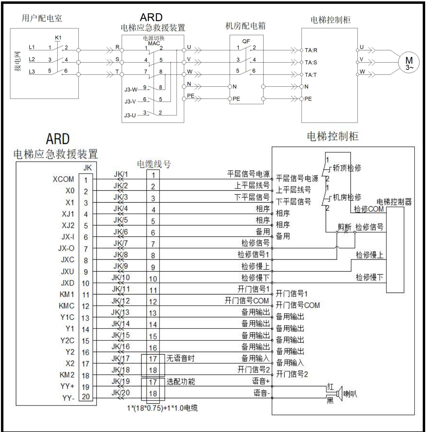
(ARD 连线图)
